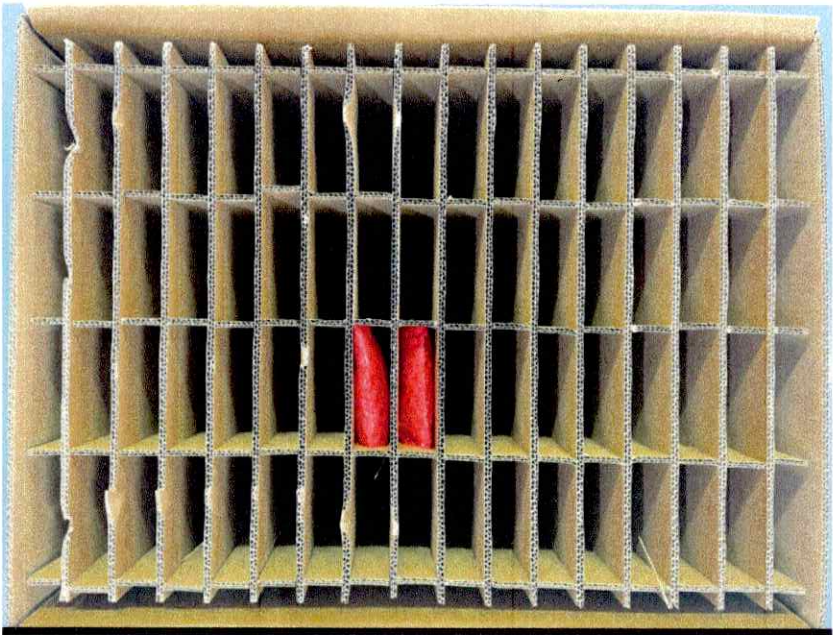
图三, 将 PA3022 按照每层 60 个, 每箱一层的方式进行包装, 同时在底层和顶部各放一块隔板, 共 2 块隔板。
