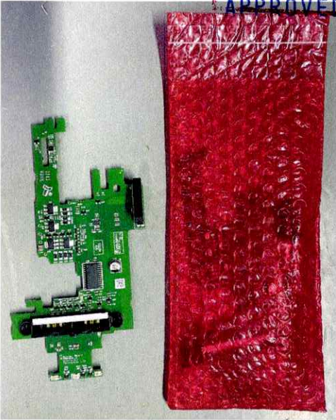
图二, 将 1 个 PA3022 如图装入气泡袋, 折叠好并粘住, 然后装入单元格内。
